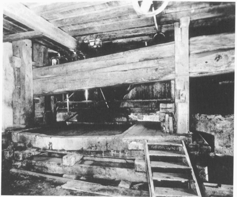
Trotte: eine Traubenpresse. Der Eichenbalken presst die Trauben durch sein Eigen- gewicht aus (undatiert)
