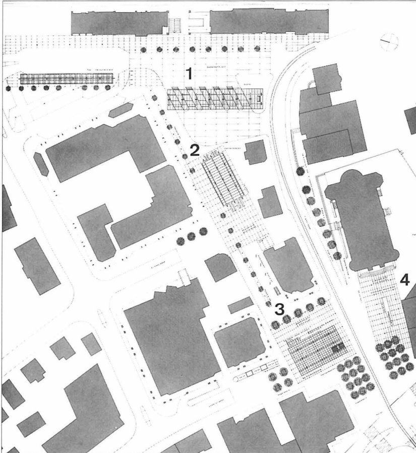
Plan des gesamten Zentrumsprojekts von Ueli Zbindens: 1: Bahnhofplatz mit dem bereits bestehenden Bushof und dem Taxisstand. 2: Veloparkhaus (bestehend). 3: Marktplatz mit multifunktionaler Markthalle (geplant). 4: Kirchplatz. Eine wichtige Funktion in der Verbindung dieser Räume kommt der Begrünung mit Pappeln und andern Bäumen sowie der Verwendung des Baumaterials zu.
